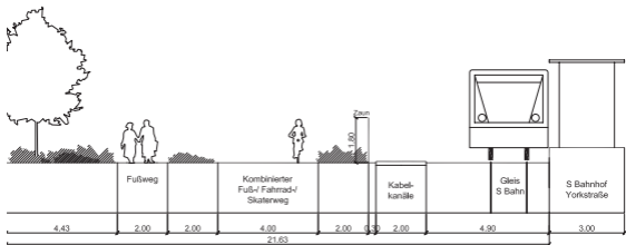
Schnitt Höhe S-Bahnhof Yorkstraße/ Platz Großgörschenstraße - Planung
