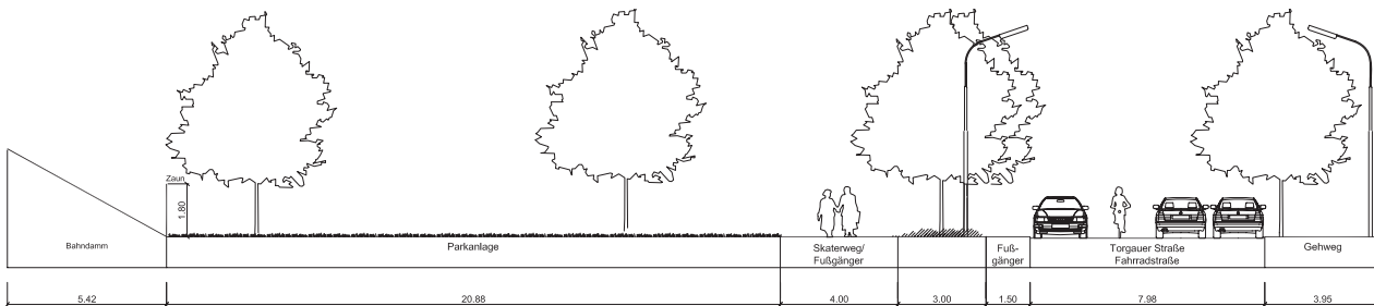
Prinzipschnitt Torgauer Straße - Fahrradstraße
