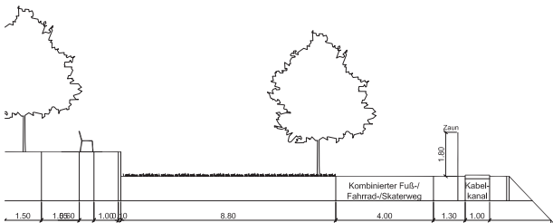
Schnitt Wannseebahngraben - Planung
